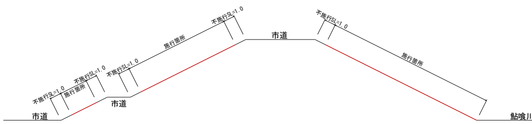
標準断面図
